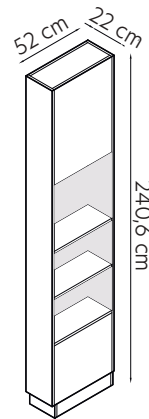
Element nr 4P Regał boczny 22 prawy
