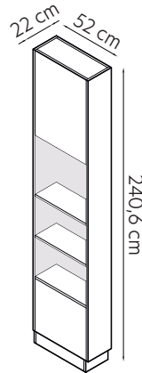
Element nr 4L Regał boczny 22 lewy
