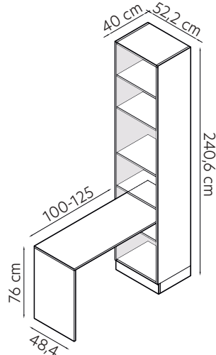
Element nr 25 Regał 52 z biurkiem
