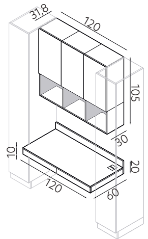
Element nr 6 Biurko podwieszane 120
